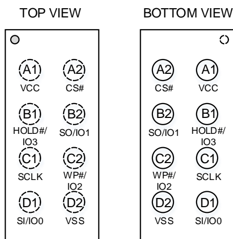
WLCSP
